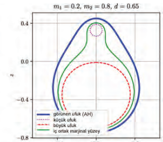
(b) İç ortak MOTS ve AH, d mesafesi azaldıkça birbirlerinden hızla uzaklaşıyor. Bu safhada her kara deliğin kendi marjinal yüzeyi bozulmadan kalıyor.
