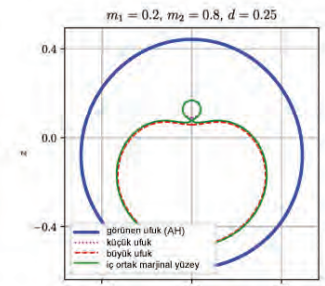
(d) İç ortak MOTS ve büyük MOTS son derece bozulmuş hale geliyor. İç ortak MOTS yıldız şeklini kaybetmiş. Küçük MOTS bir bariyer görevi görüyor ve birleşmeyi engelliyor.
