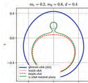
(c) d mesafesi daha da azalıyor ve iç ortak MOTS bozulmaya başlarken AH göttükçe daha yuvarlak bir şekil alıyor. Büyük marjinal yüzeyde de bozulma görülmüyor.
