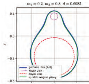
(a) Ortak MOTS oluşumundan hemen sonra farklı marjinal yüzeyler. Bu ayrılmada iç ortak MOTS ve AH birbirlerine son derece yakın.
