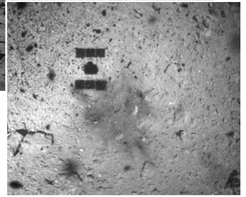
22 Şubat 2019'da JAXA tarafından yayımlanan bu fotoğraf, Hayabusa2 uzay aracının Ryugu asteroidi üzerine düşen gölgesini gösteriyor.
